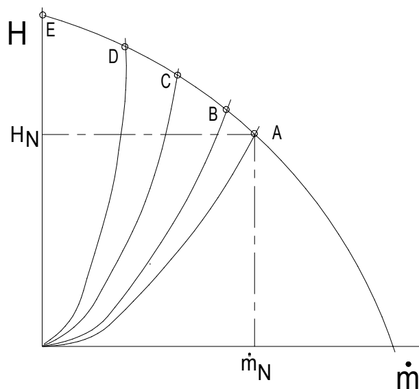
Рабочая точка на характеристике сети трубопроводов и характеристической кривой насоса
