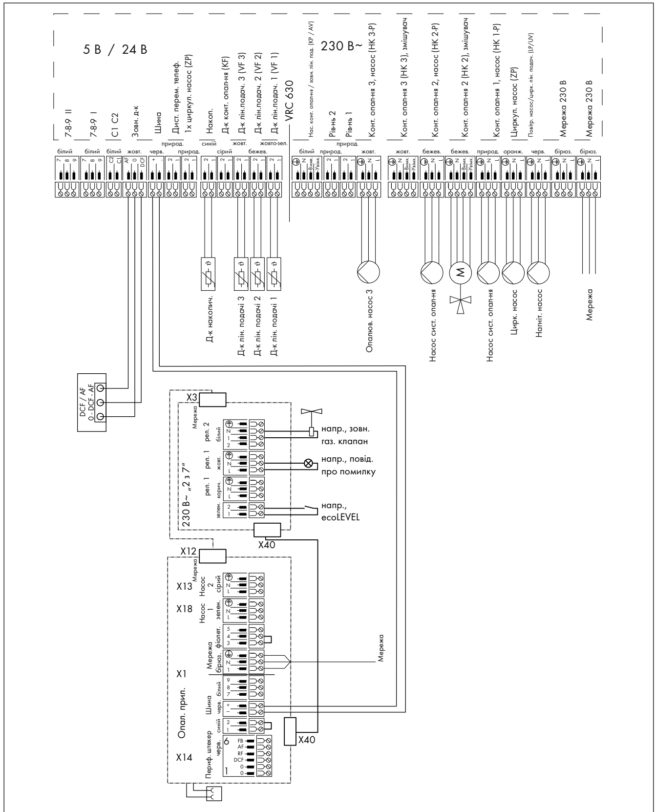
Мал. 5.15 Підключення регулювального приладу VRS 620 або VRC 630
