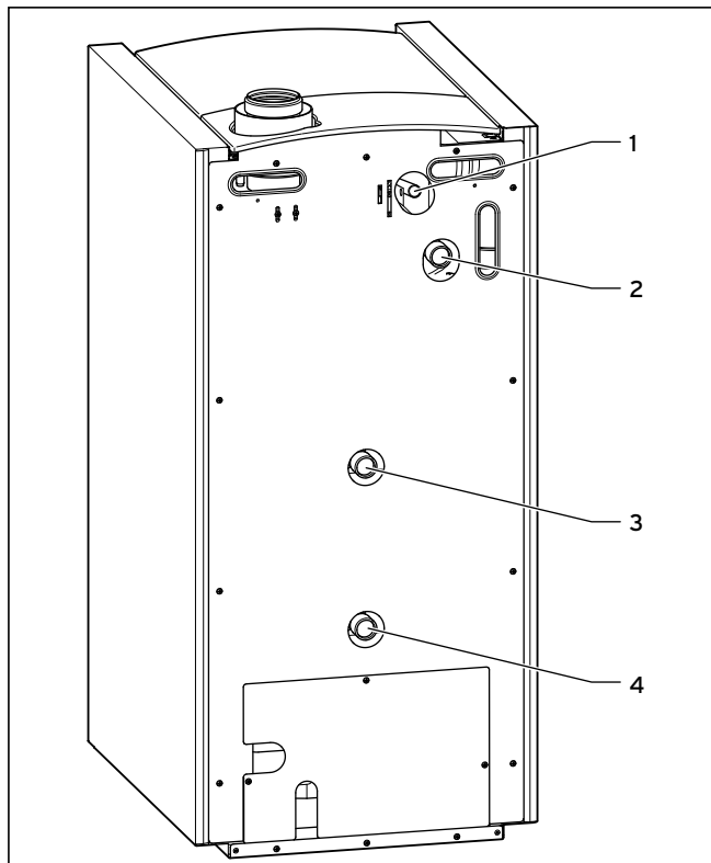
Мал. 5.4 Підключення опалення
