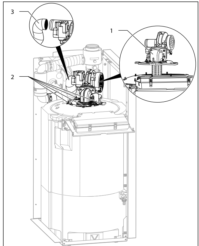
Мал. 8.1 Демонтаж пальника
