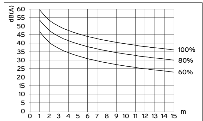
Мал. 6.3 Рівень звукового тиску зовнішнього модуля в дБ(A) залежно від віддаленості й числа оборотів вентилятора для VWL 101/3 S при установці у вільному звуковому полі
