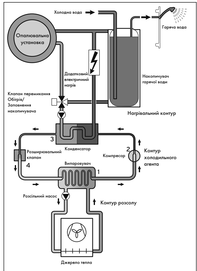
Мал. 3.4 Принцип дії теплового насоса (внутрішній модуль)
