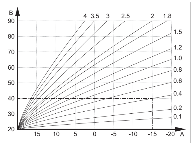
A 室外温度 °C B 供水标准温度 °C
